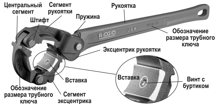
Рис. 1 – Колоночный трубный ключ
